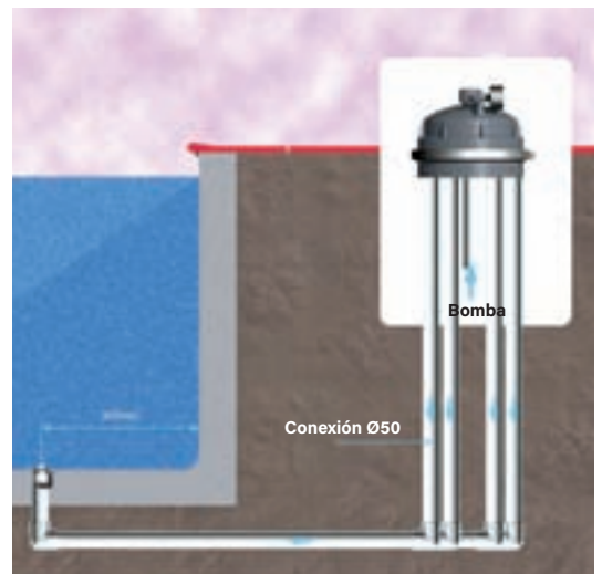
Instalación válvula Net'n'Clean
