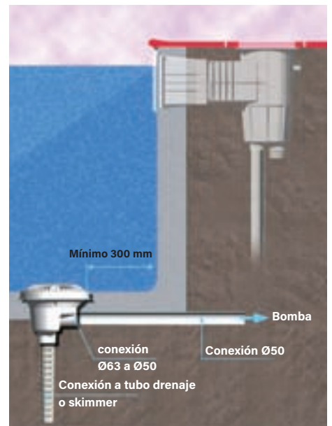
Instalación sumidero
